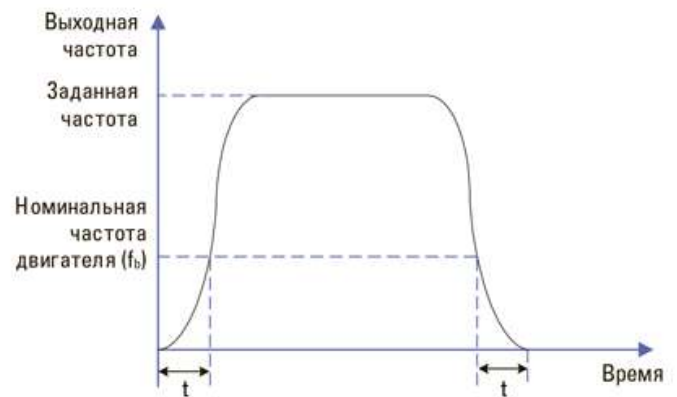
Картина В: схема S-кривой ускорения/торможения В
