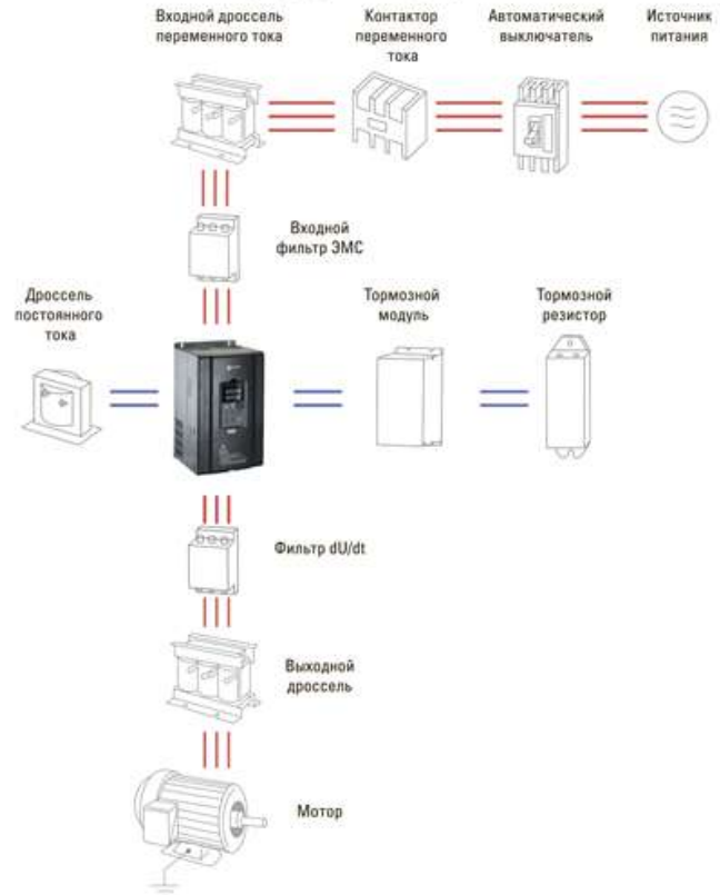
Рис. 11-1 Схема подключения периферийных устройств
