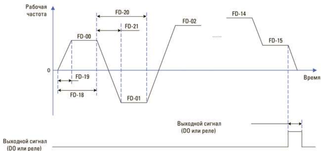
Схема работы простого ПЛК
