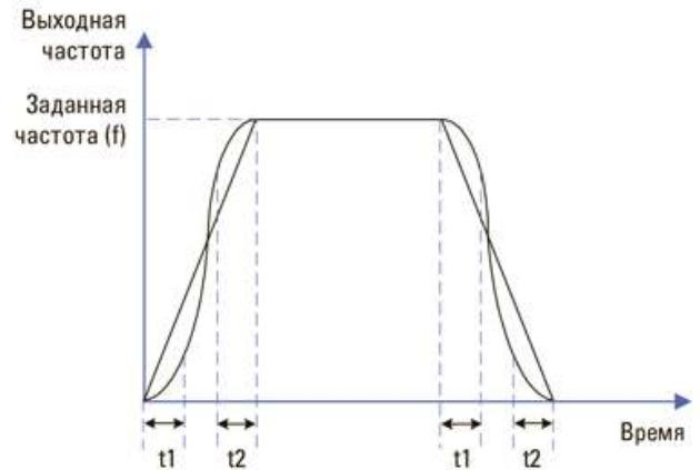
Картина А: схема S-кривой ускорения/торможения А
