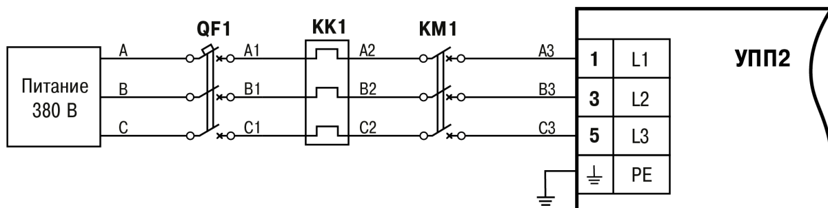
Рисунок 5.4 – Схема подключения питания
