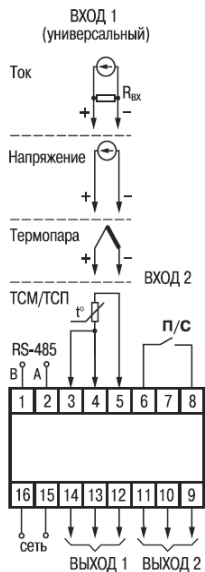
Рисунок Б.1 – Общая схема подключения
