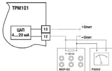
Рисунок Ж.4 – Подключение ВУ1 вида И
